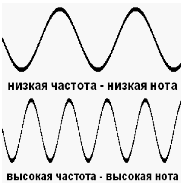
Рис. 3.1. Звуковые волны
