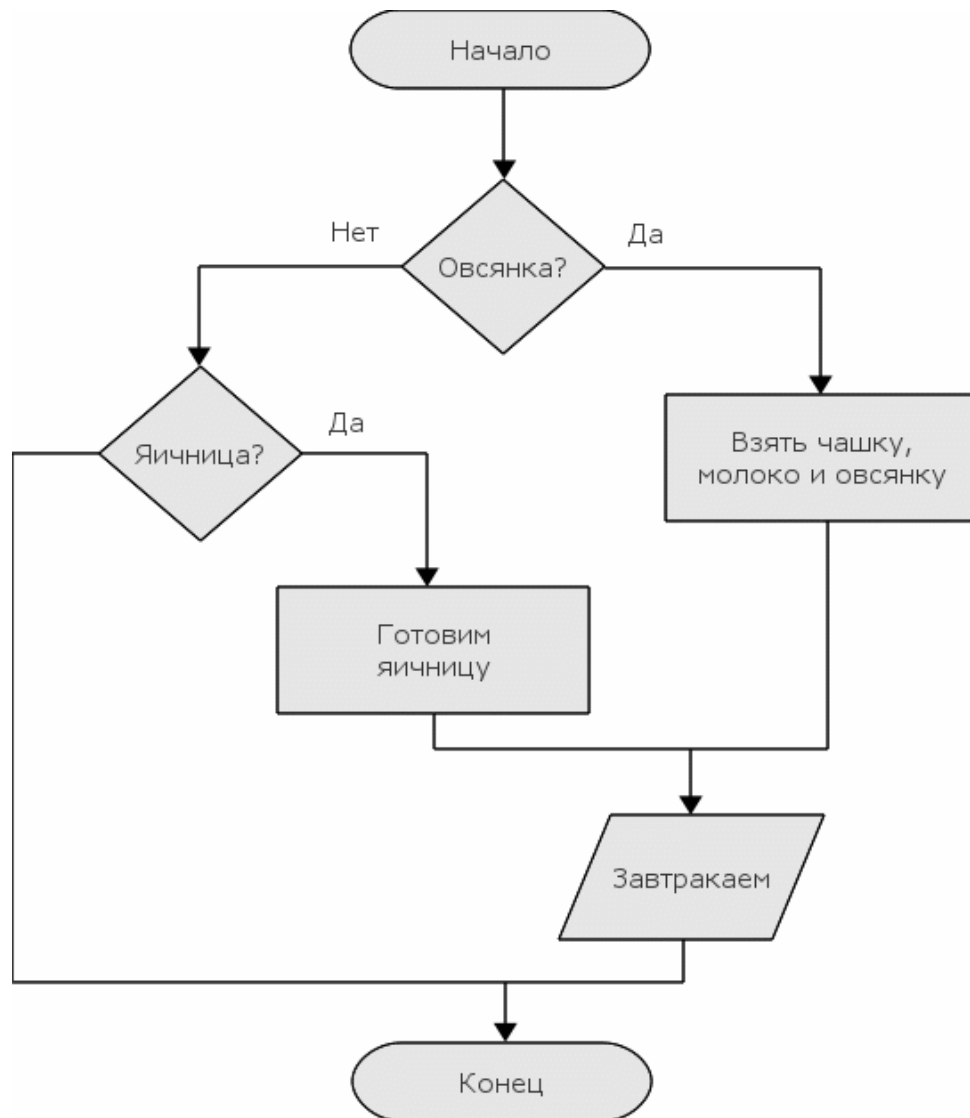
Рис. 4.2. Завтрак — блок-схема
