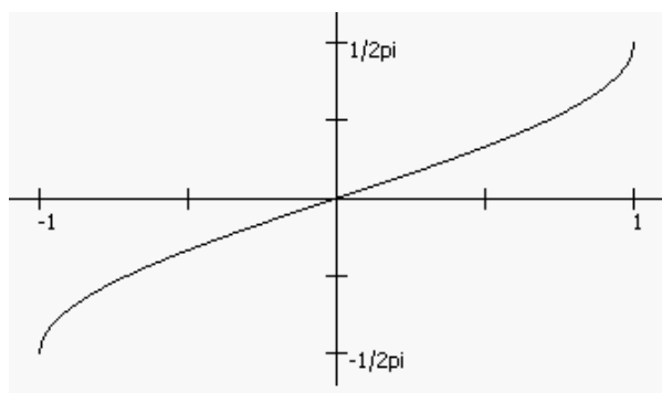
Рис. 14.6. Функция \text{asin}()
