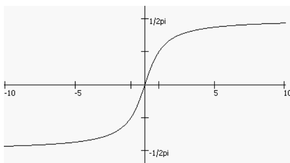
Рис. 14.7. Функция \text{atan}()
