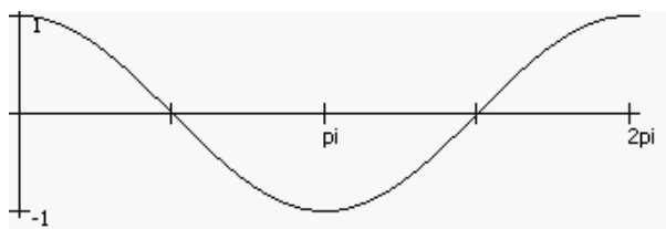
Рис. 14.2. Функция \cos()
