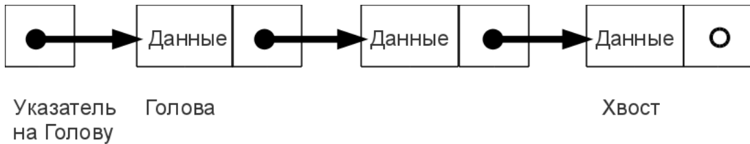
Рис. 17.3. Связный список
