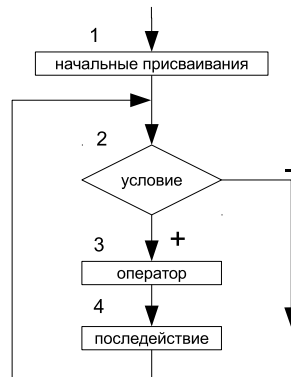
Рис. 3.22: Алгоритм работы цикла с параметром
