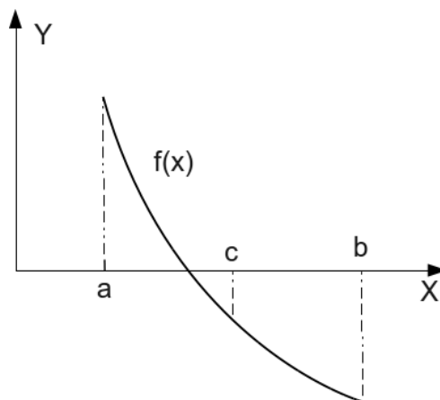
Рис. 4.3: Графическая интерпретация метода половинного деления
